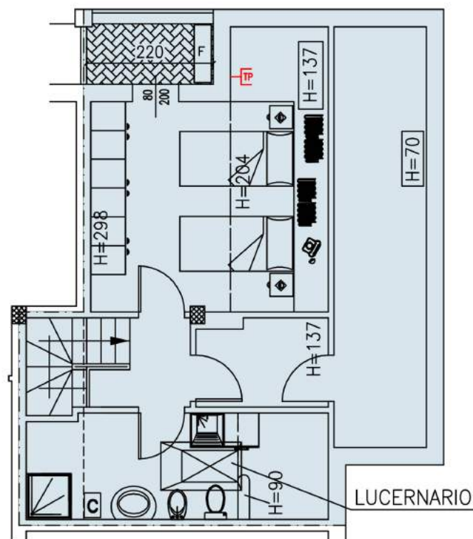
PIANTA PIANO SOTTOTETTO 1:100
