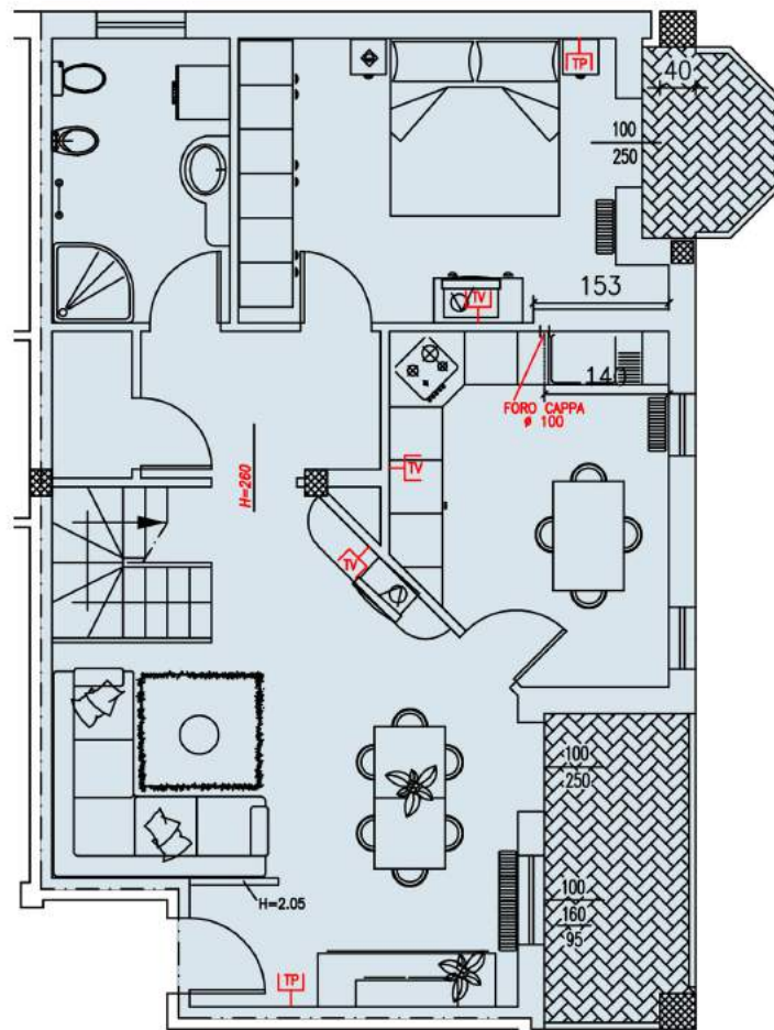
PIANTA PIANO SECONDO 1:100
